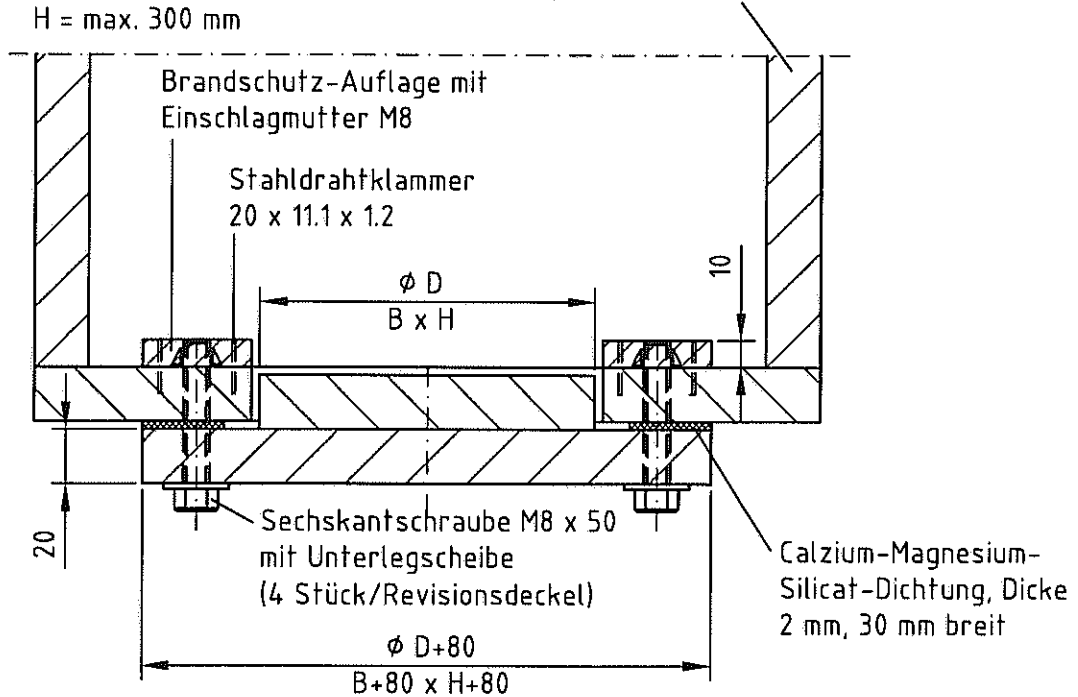
Revisionsöffnung werkseitig vormontiert
