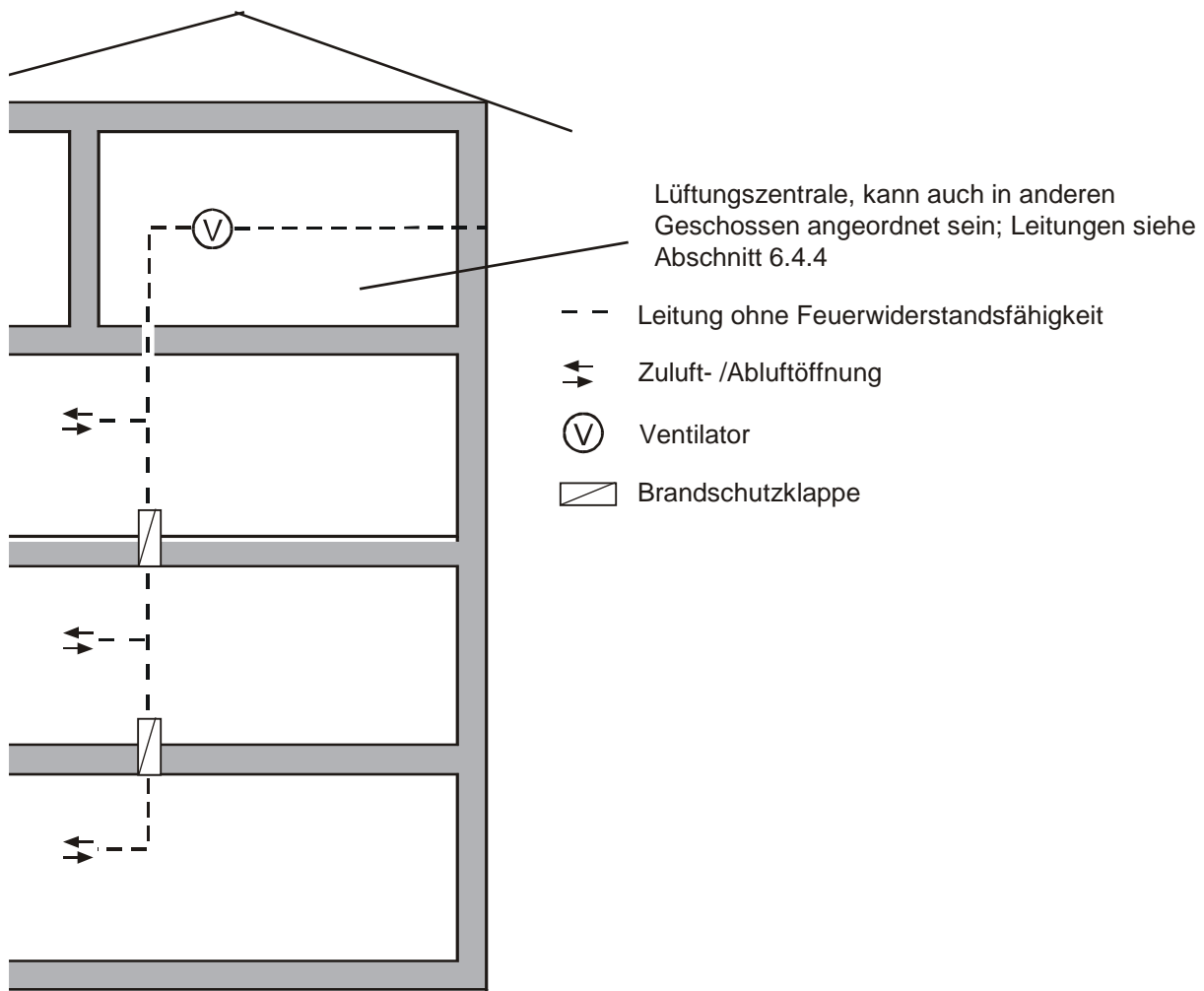
Brandschutzklappen an den Durchdringungsstellen der feuerwiderstandsfähigen Decken
